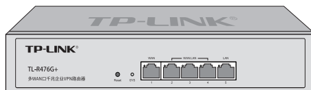
图1-6 TL-R476G+前面板示意图
